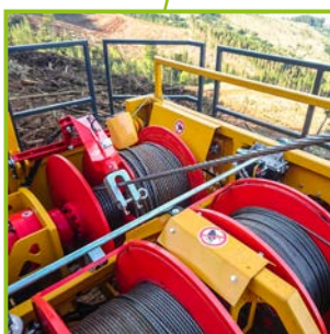
ÜBERSICHTLICHE WINDENEINHEIT
